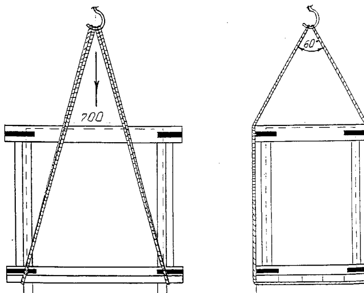
Рис. 10 Схема строповки.
