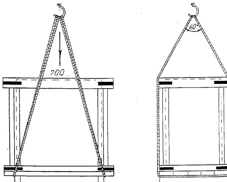
Рис. 10 Схема строповки
