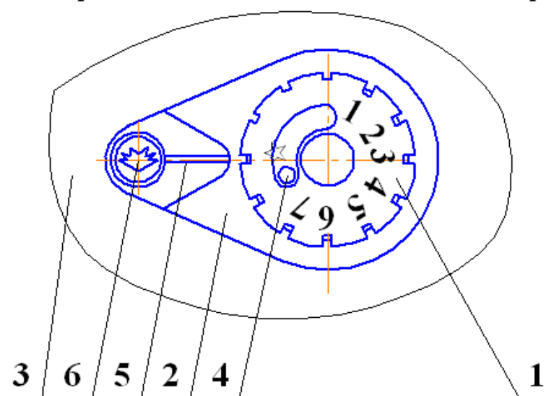
Рис.4 Элементы управления газовым клапаном (вид сверху).
