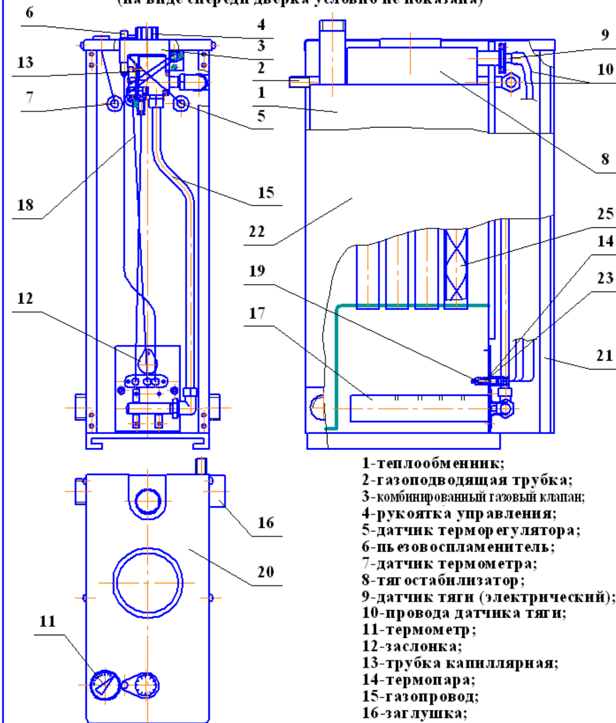
Рис.1 Конструкция аппарата
