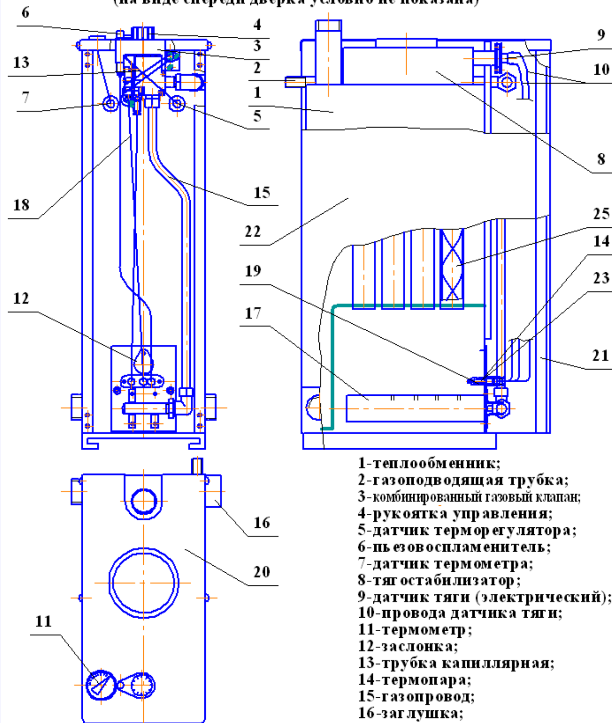
Рис.1 Конструкция аппарата
