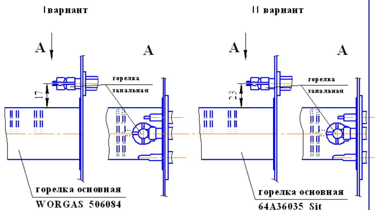
Рис.8 Схема расположения горелки запальной относительно основной.
