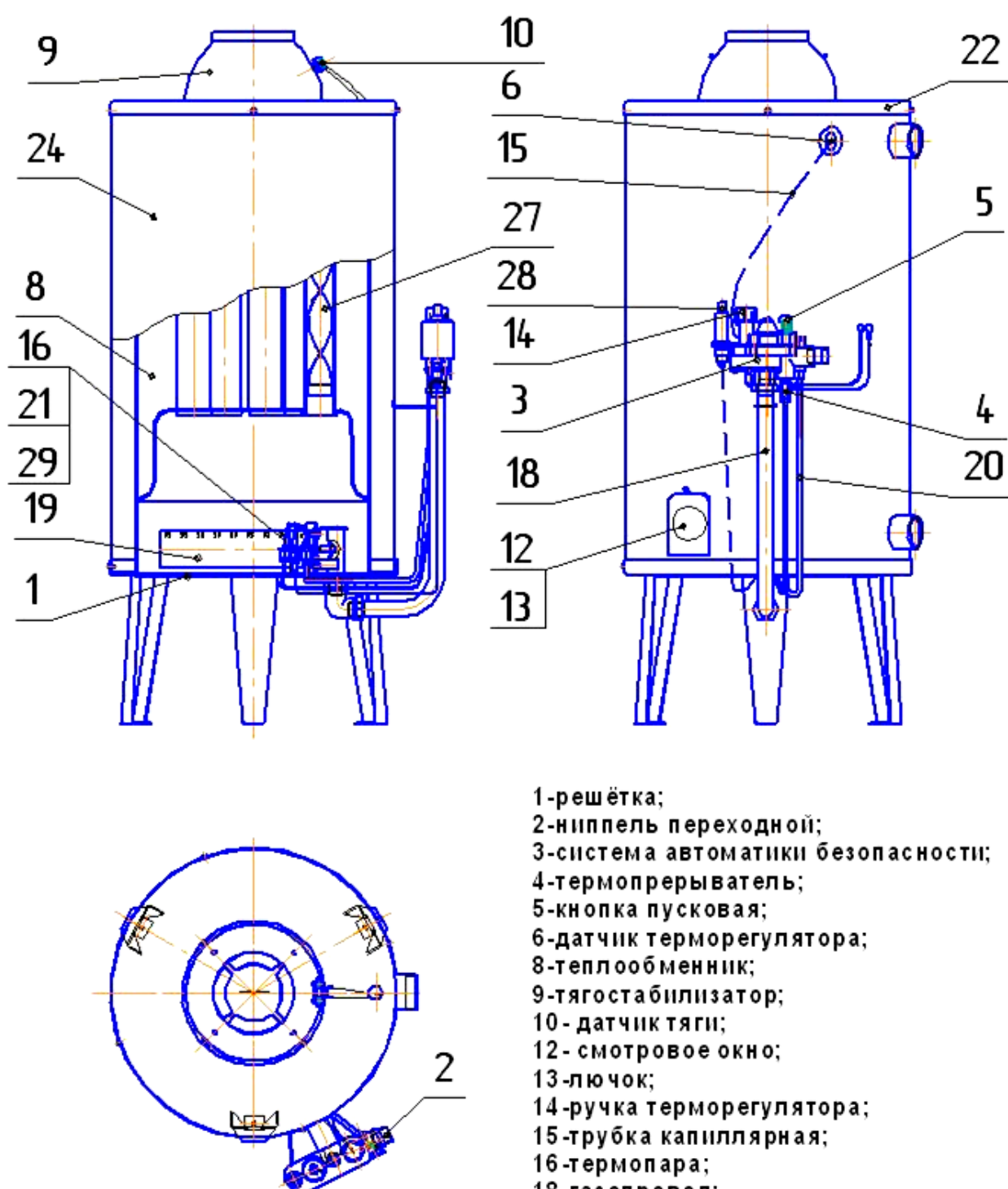
Рис.1 Конструкция аппарата.
