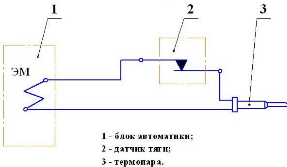
Рис.3 Схема электрическая.
