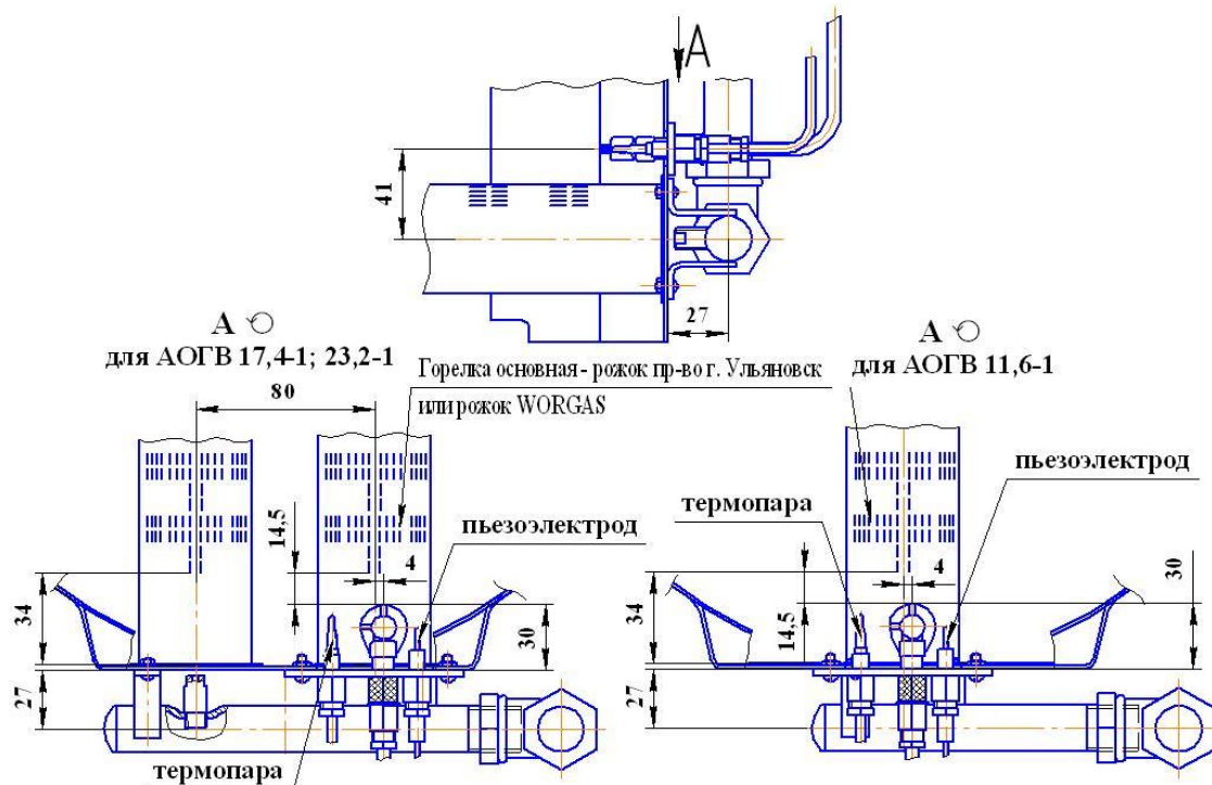
Рис.7б Схема расположения горелки запальной относительно основной (рожковой) (см. таблицу пункт 4А, вариант III).
