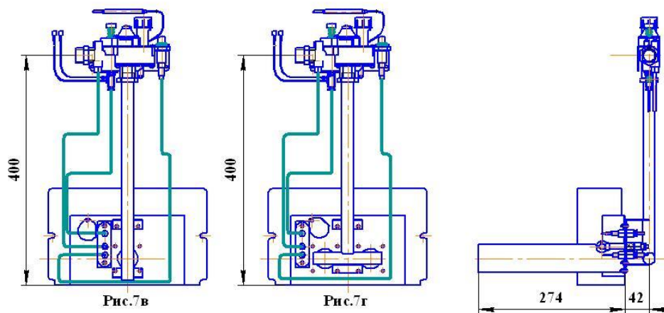
Рис.7в,г. Схема газогорелочного устройства с рожковыми горелками - УГ-САБК-АТ (см. табл. п. 4А, вариант IV)
