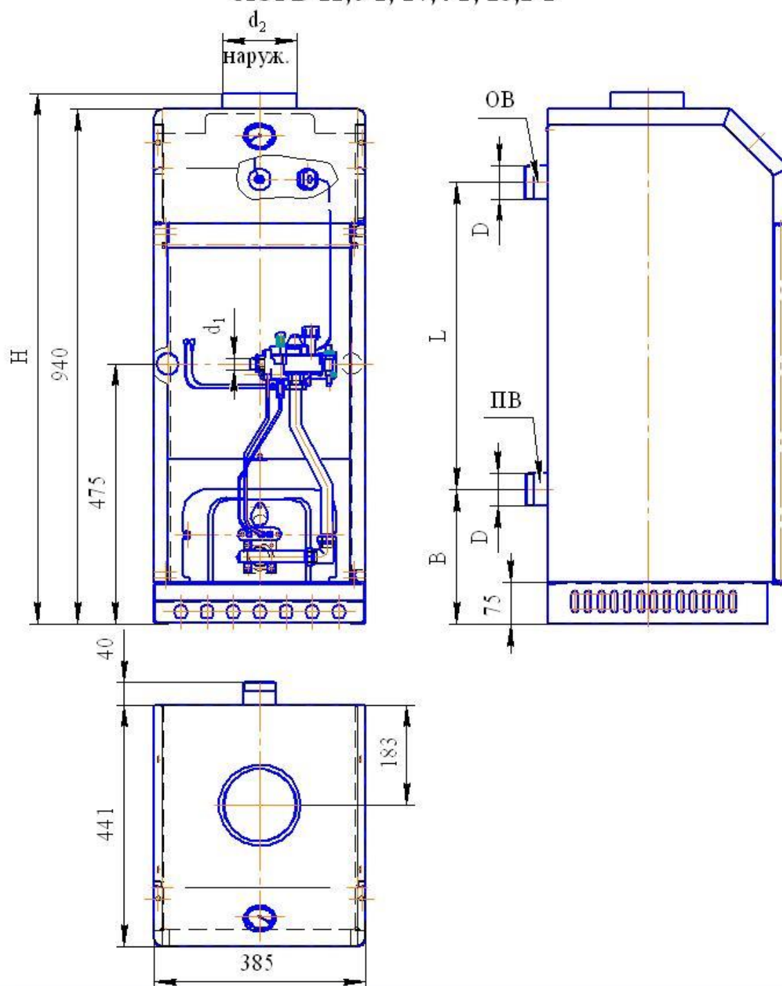
Рис.2 Габаритные и присоединительные размеры аппаратов АОГВ-11,6-1; 17,4-1; 23,2-1
