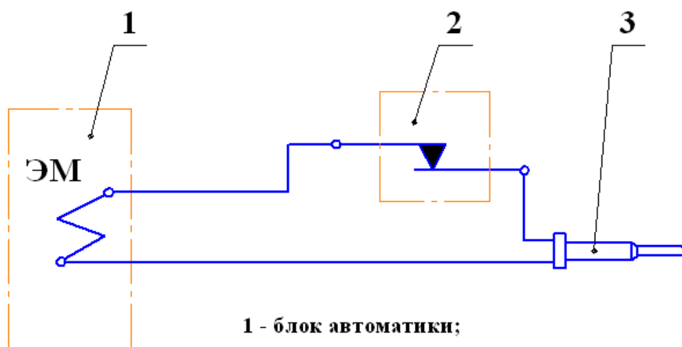
Рис.3 Схема электрическая.
