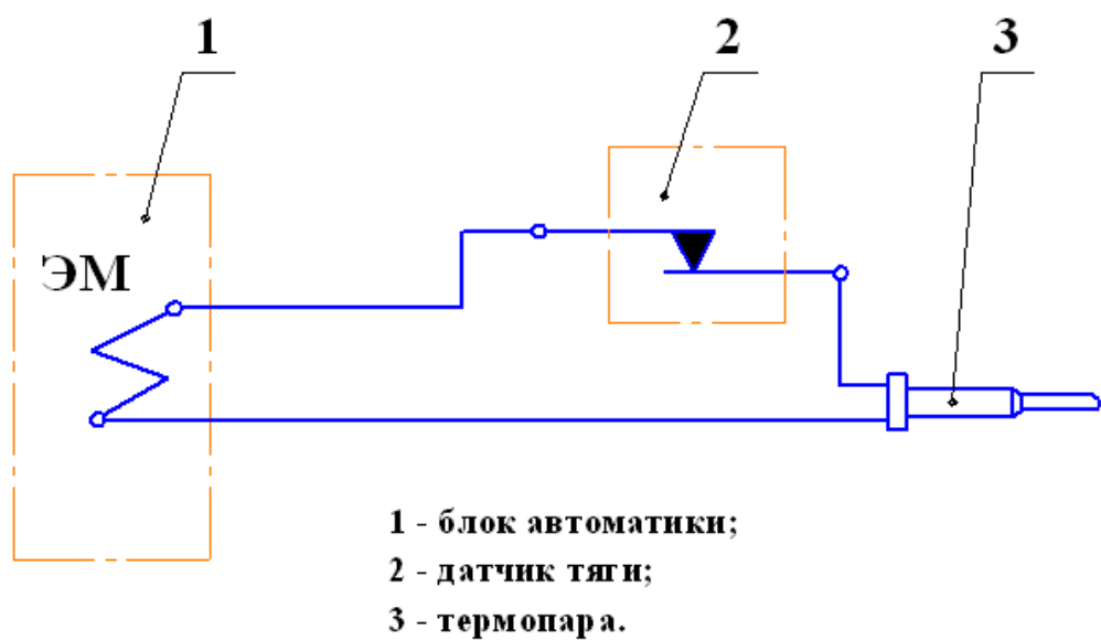
Рис.3 Схема электрическая.
