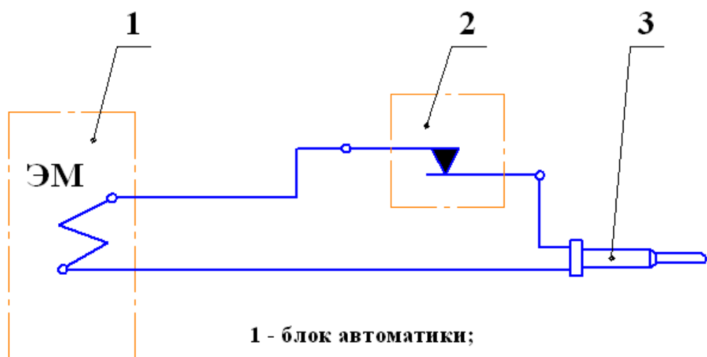
Рис.3 Схема электрическая.
