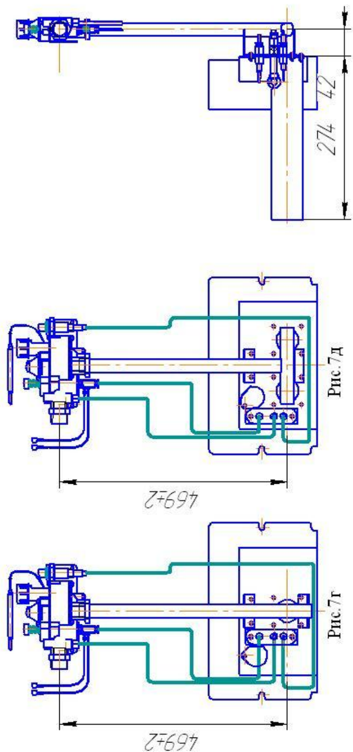
Схема газогорелочного устройства с рожковыми горелками - УГ-САБК-АТ (см. табл. п. 4А, вариант V)
