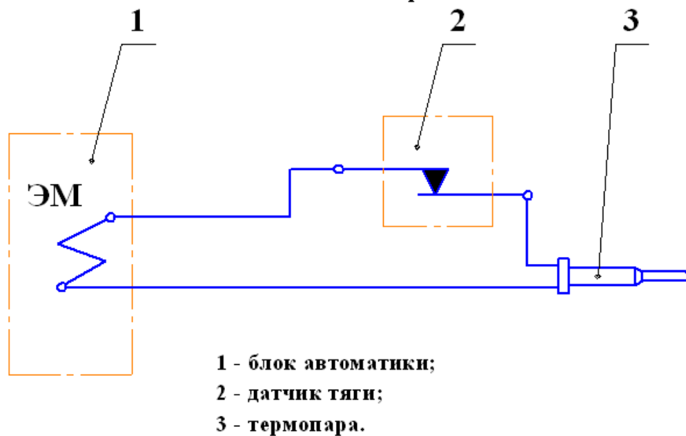
Рис.3 Схема электрическая.
