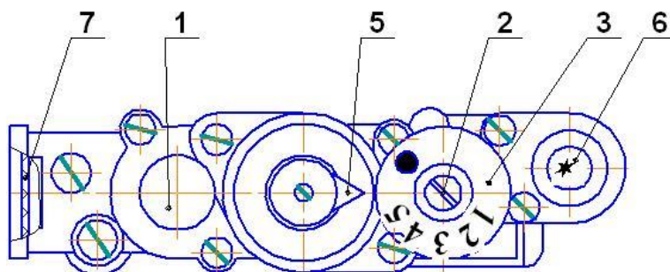
Рис.4 Элементы управления блока автоматики. Вид сверху
