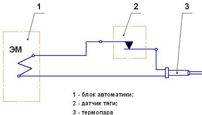
Рис.3 Схема электрическая
