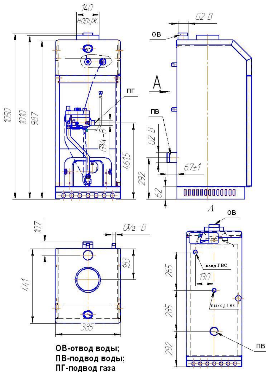
Рис.2 Габаритные и присоединительные размеры аппарата АКГВ 29-1
