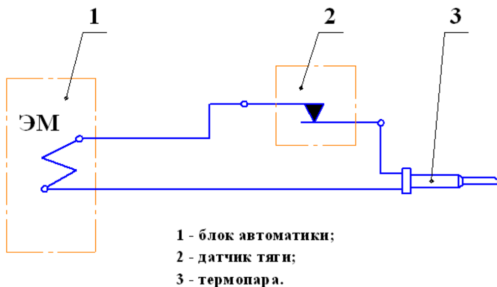
Рис.3 Схема электрическая.
