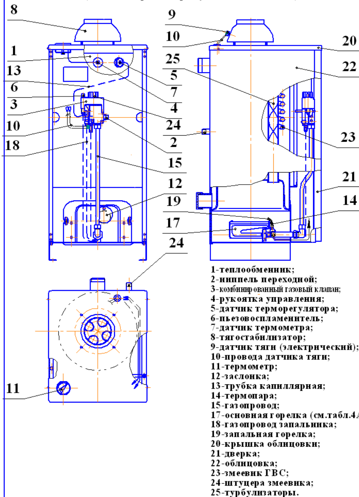
Рис.1 Конструкция аппарата (на виде спереди дверка условно не показана)
