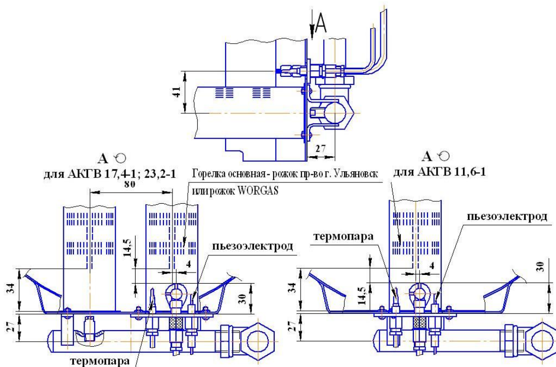
Рис. 7б Схема расположения горелки запальной относительно основной (рожковой) (см. таблицу пункт 4А, вариант III).
