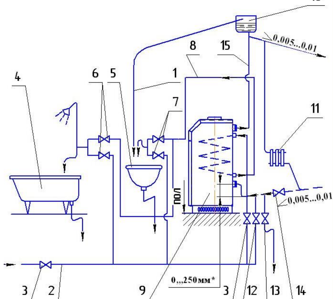
Рис.6 Примерная схема установки аппарата АКГВ
